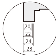
A 詳細図
