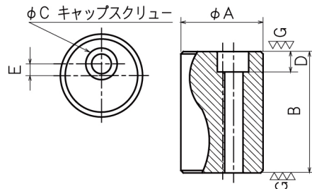
(寸法表) 単位 長さ(mm) 質量約(g)
