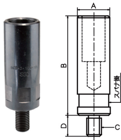
(寸法表)
